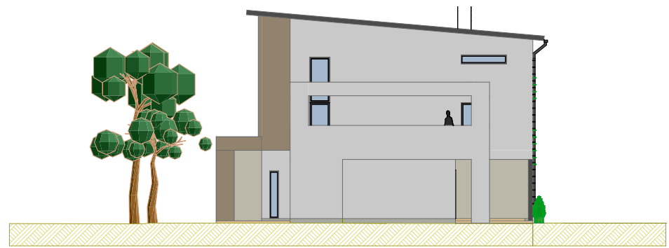
Julkisivu länteen
