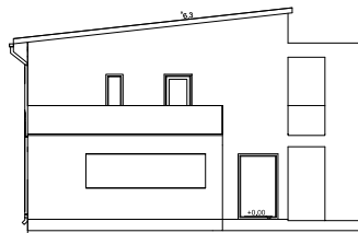
JULKISIVU POHJOISEEN
