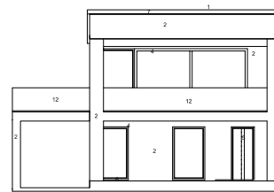
JULKISIVU ITÄÄN
