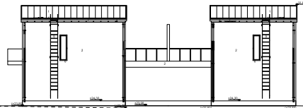
JULKISIVU LÖUNÄISEEN
