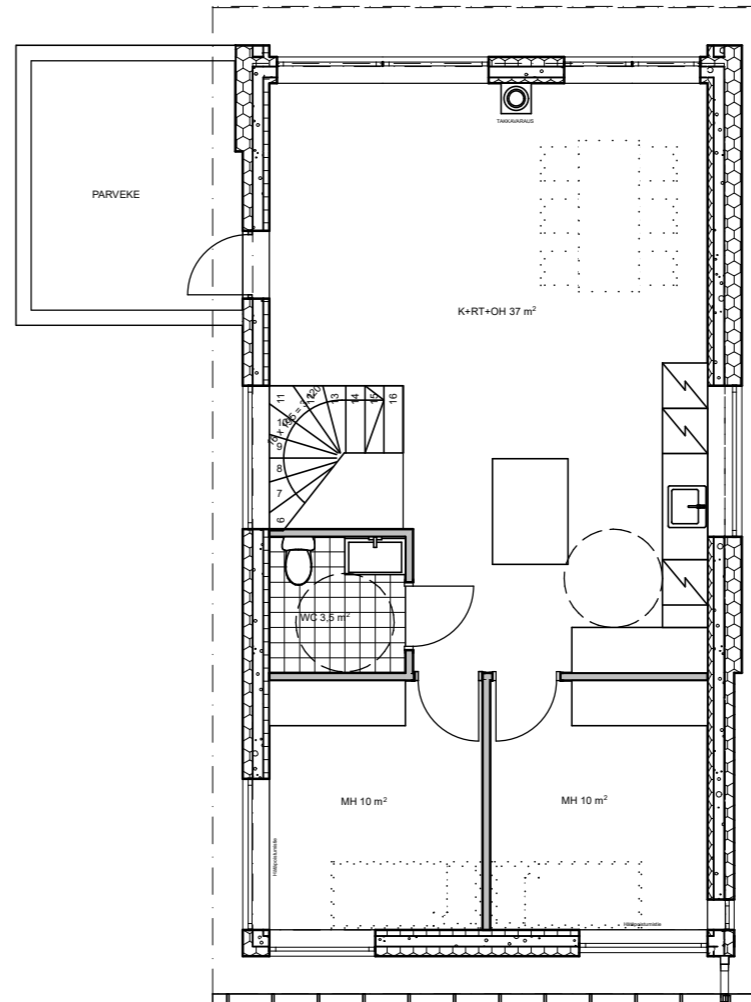
2.krs
